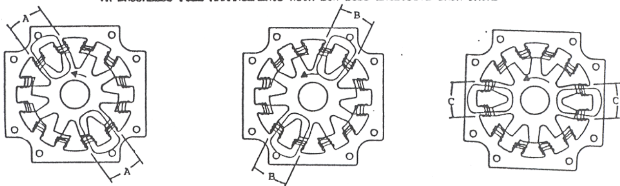
FIG. 7B 12/10 3 PHASE
